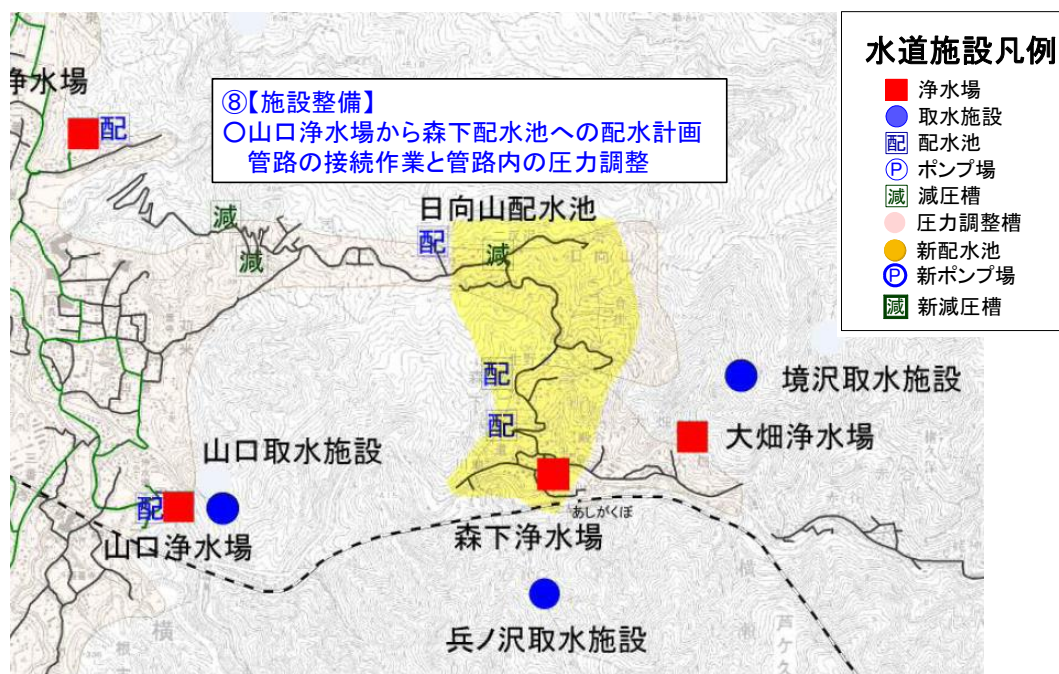
図 2-10 山口浄水場から森下地区への配水計画の概要
