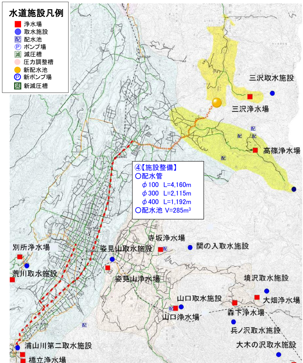
図 2-6 新三沢配水池への配水計画の概要
