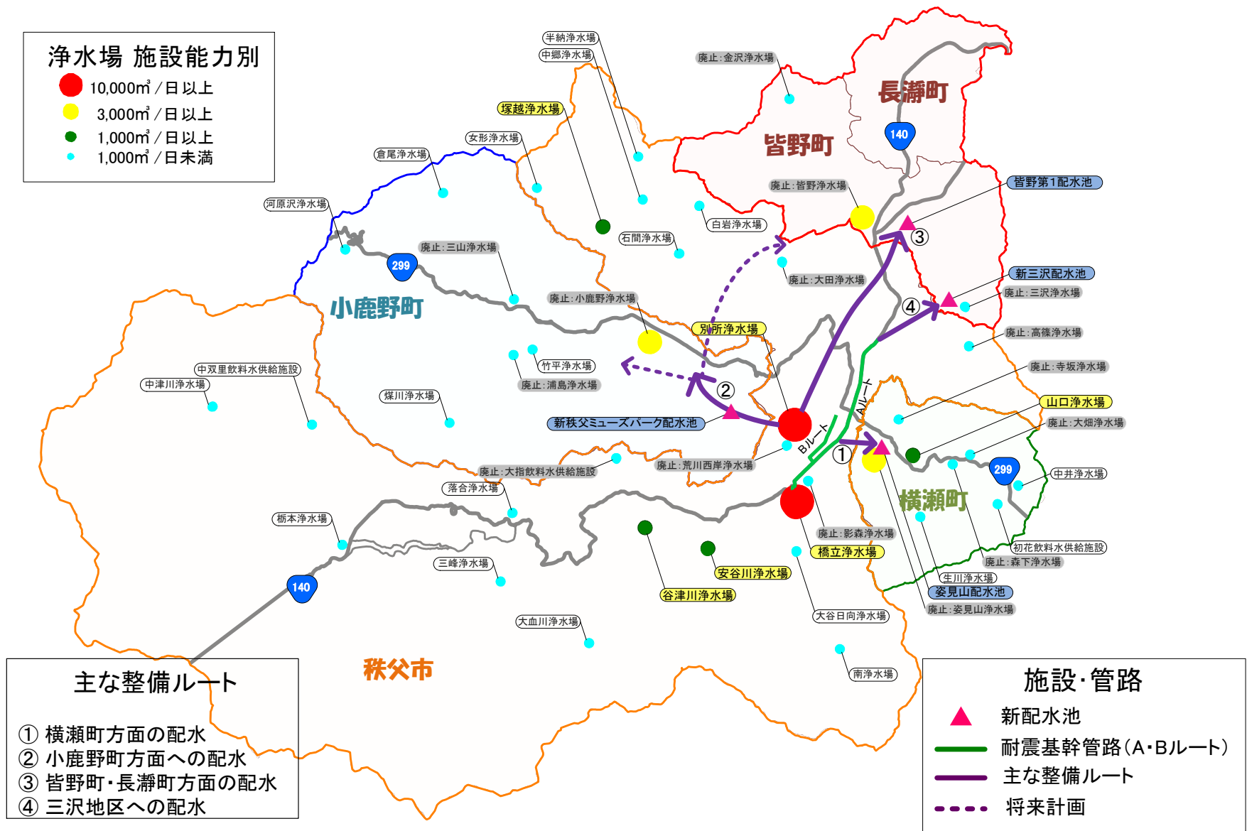
図 2-1 秩父地域の水道施設整備計画
