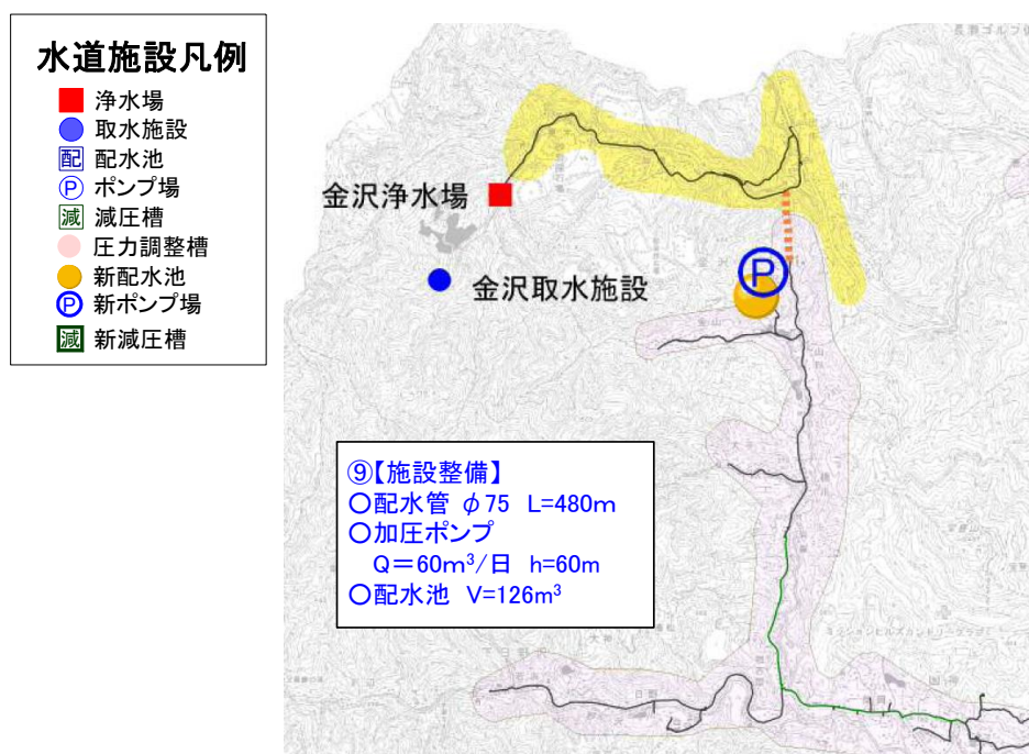
図 2-11 皆野第1配水池から金沢浄水場エリアへの配水計画の概要
