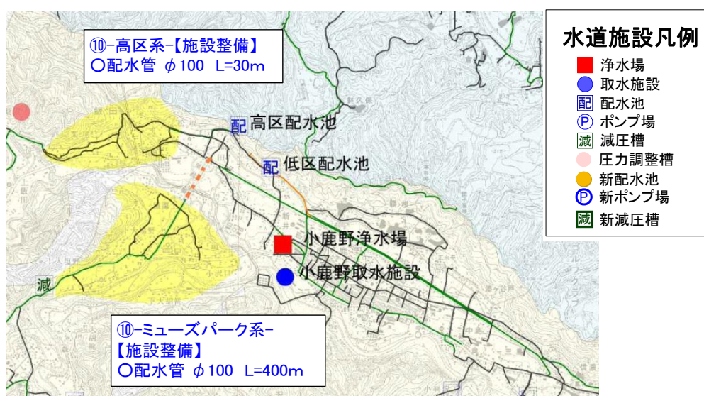
図 2-12 小鹿野浄水場エリアの拡大（竹平浄水場エリア・三山浄水場エリアへの配水）の概要
