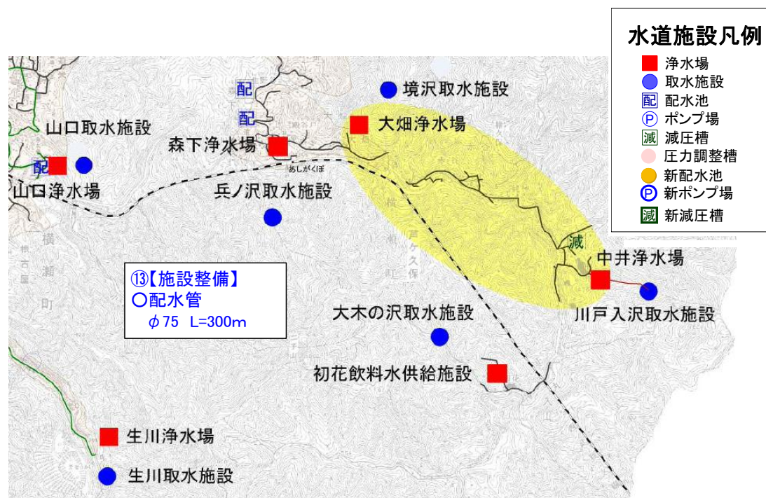
図 2-15 中井浄水場から大畑浄水場エリアへの配水計画の概要
