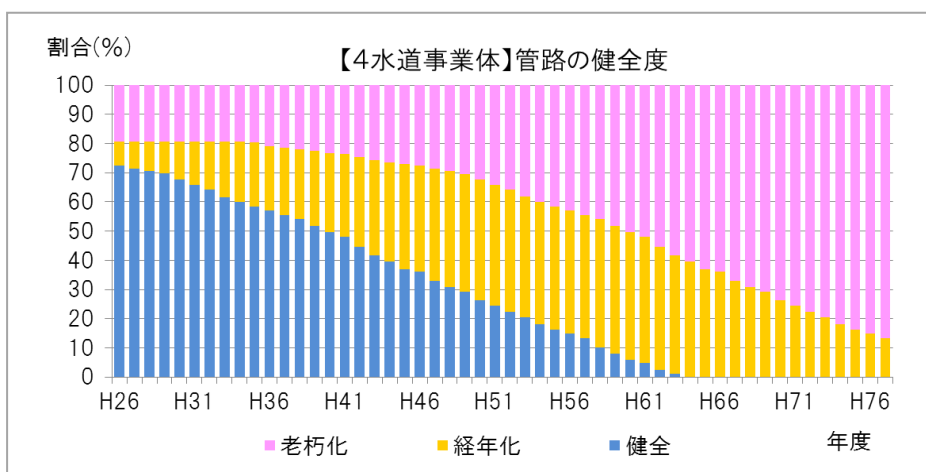
図 2-17 管路の健全性の推移
