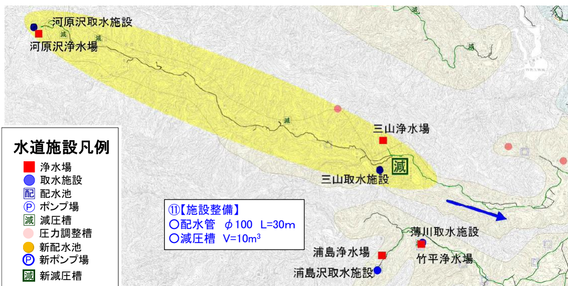
図 2-15 河原沢浄水場エリアの拡大（三山地区への配水）の概要
