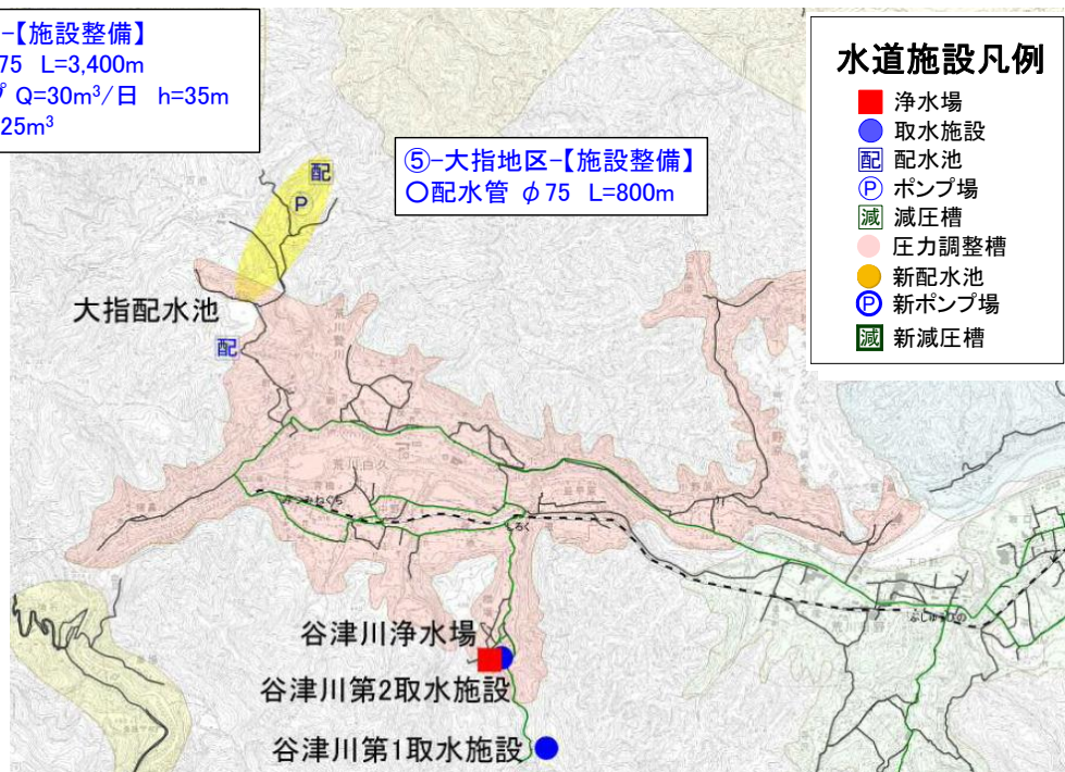
図 2-7 大指地区、古池地区（未給水地区）への供給計画の概要
