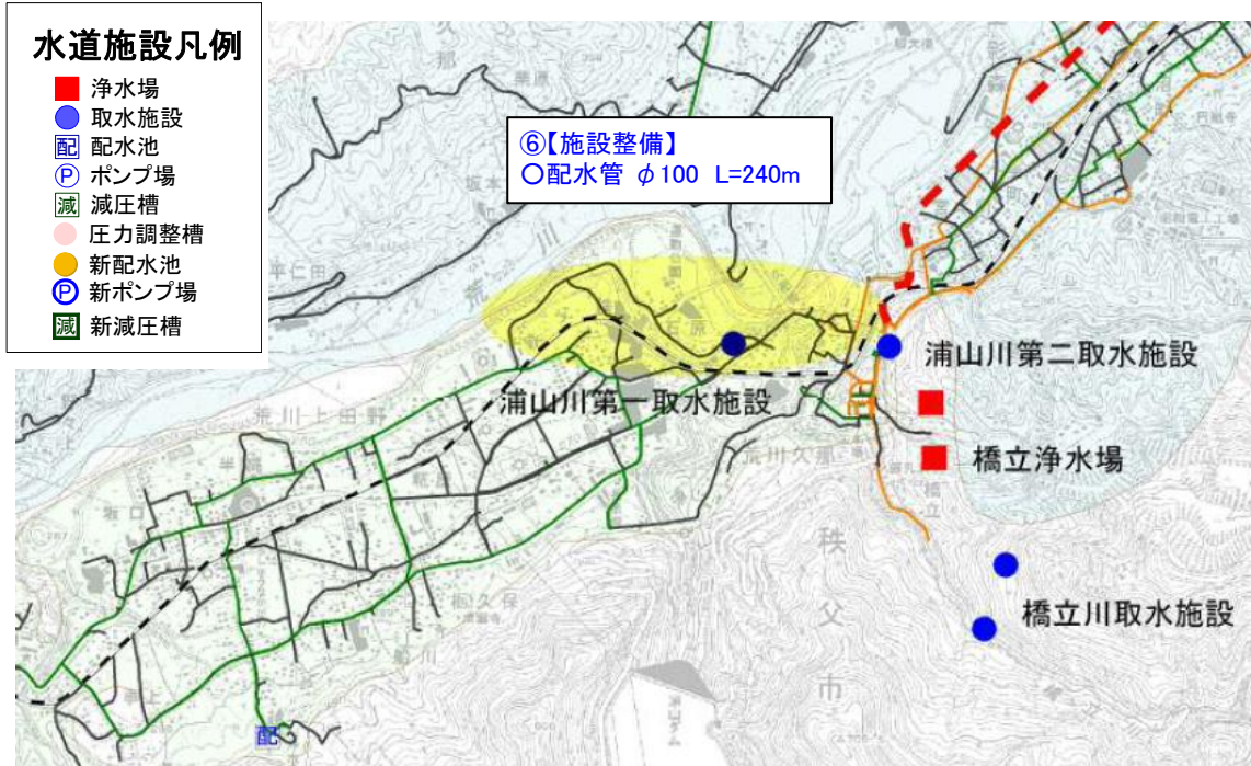
図 2-8 石原地区への配水計画の概要
