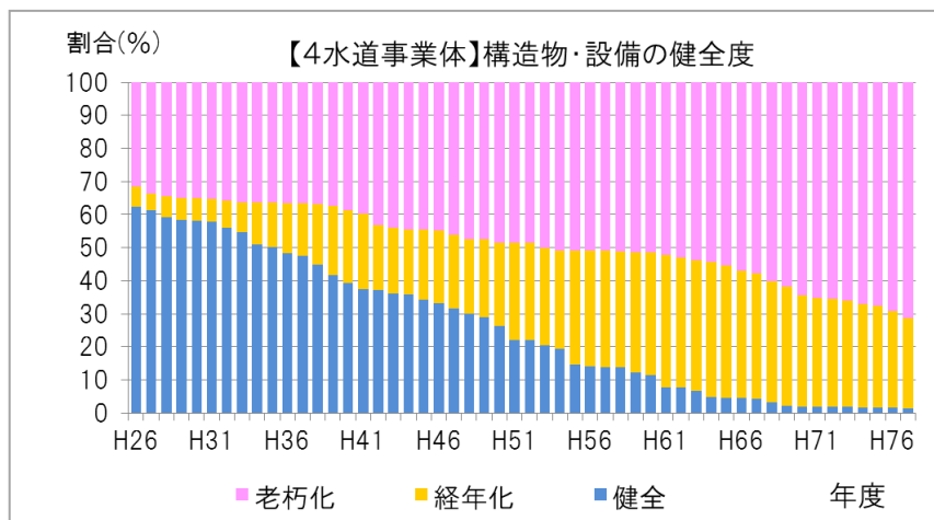
図 2-16 構造物・設備の健全性の推移
