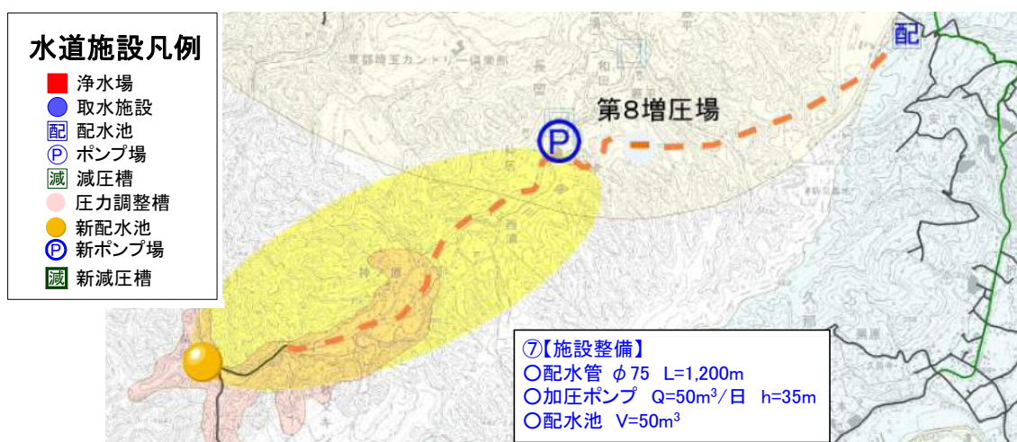
図 2-9 新秩父ミュージックパーク配水池から長留地区、柴原地区への配水計画の概要
