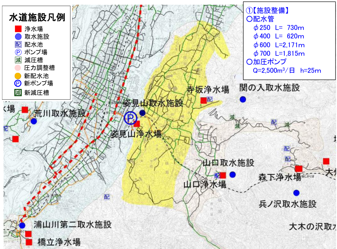
図 2-2 姿見山配水池への配水計画の概要
