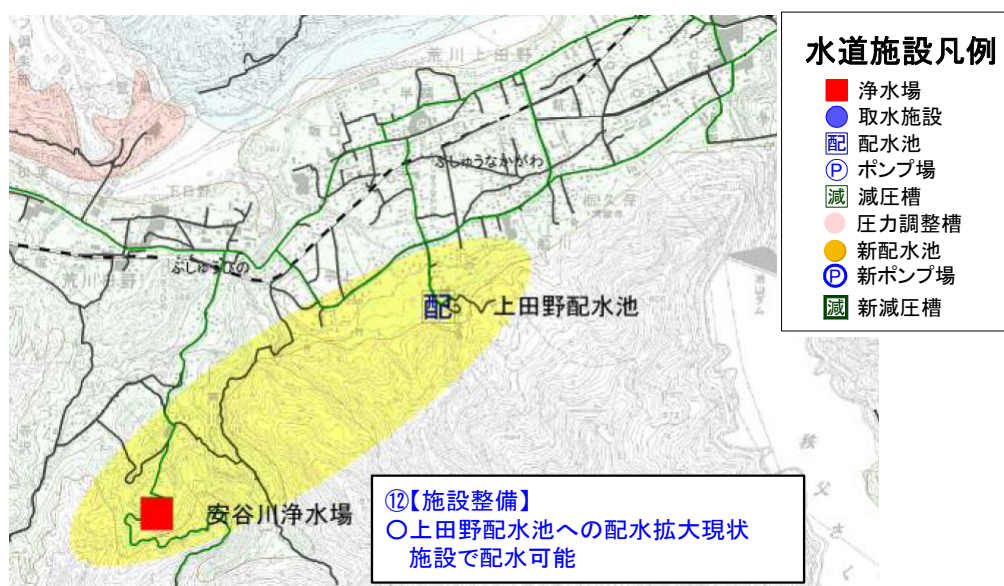
図 2-14 上田野配水池及び橋立浄水場への配水計画の概要
