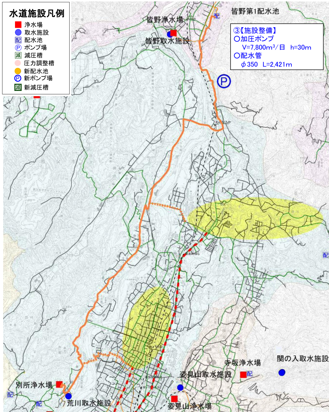
図 2-5 皆野第1配水池への配水拡大の概要
